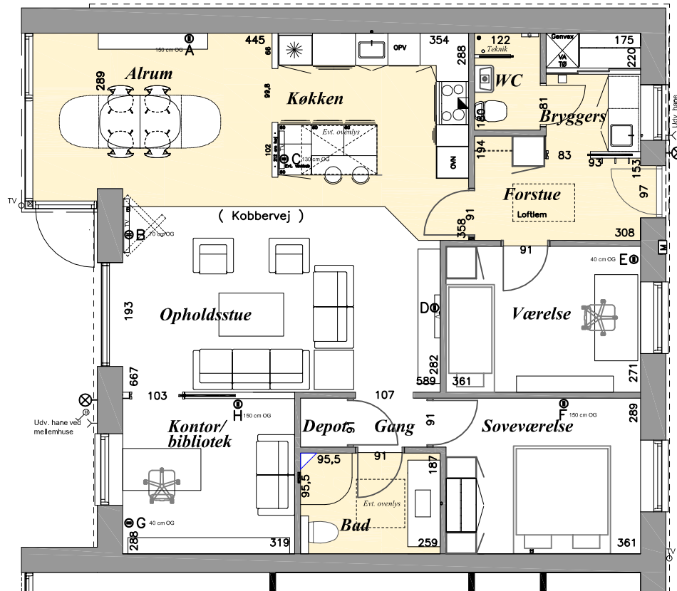
Plantype ASM 114 mål 1:100 Soveværelse, værelse, kontor og depot.
